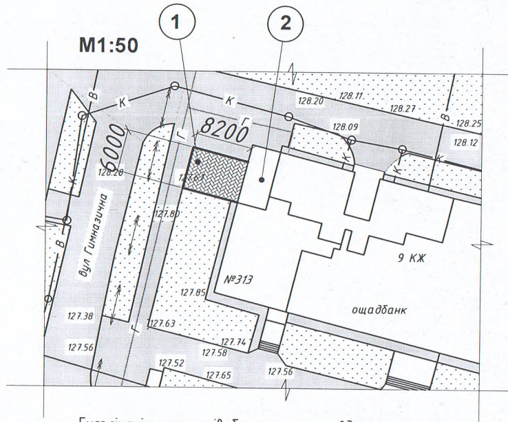
Експлікація елементів благоустрою майданчика
